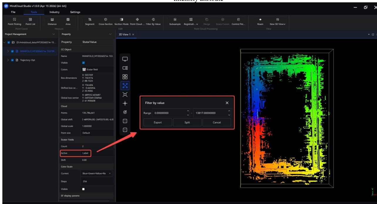
Label attribute
